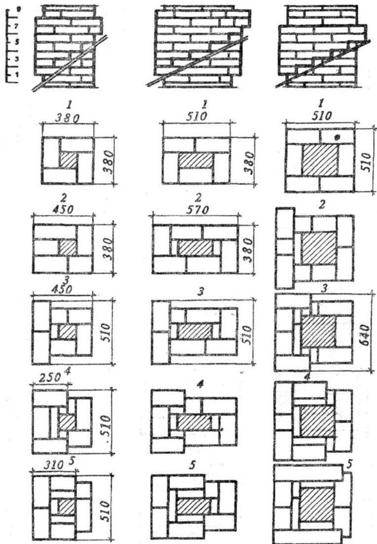
Рис. 96. Кладка выдры:
