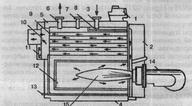
Рис. 26. Котел Logano SE: 1 - пульт управления; 2 - дверь котла; 3 - направляющий элемент водяного контура; 4 - рама котла; 5 - теплоизоляция; 6 - подающая линия котла; 7 - штуцер предохранительного клапана; 8 - обратная линия котла; 9 - композитные отопительные поверхности; 10 - сборник дымовых газов; 11 - ревизионное отверстие; 12 - камера сгорания; 13 - спуск воды из котла; 14 - горелка; 15 - пламя грелки
