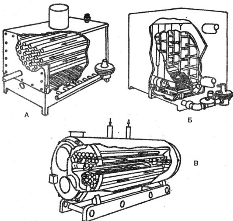
Рис. 22. Водогрейные котлы:
