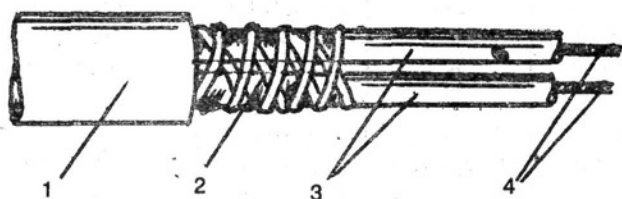
Рис. 79. Двухжильный резистивный кабель: 1 - оболочка; 2 - медный экран; 3 - изоляция из термостойкого полимера; 4 - токонесущие проводники
