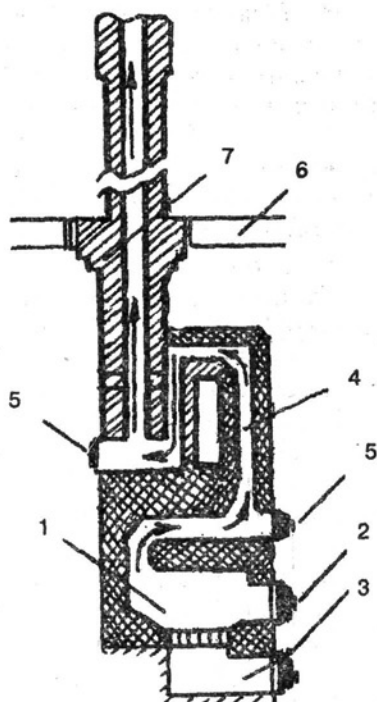
Рис. 87. Дымоход печи:
