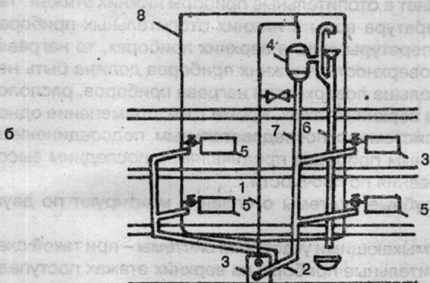
Рис. 6. Двухтрубная схема водяного отопления:
