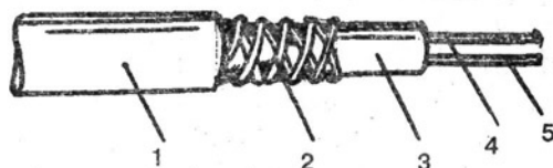
Рис. 80. Нагревательный кабель марки ЕСО: 1 - оболочка из ПВХ-пластика; 2 - оплетка из медной проволоки; 3 - теплостойкий ПВХ-пластик; 4 - вспомогательная жила из отожженной меди; 5 - нагревательная жила
