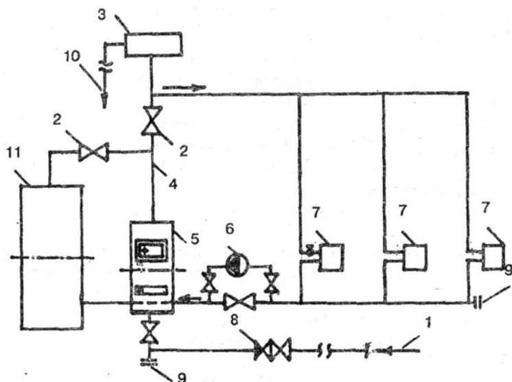
Рис. 11. Система отопления с принудительной циркуляцией теплоносителя и баком аккумулятором теплоты:
