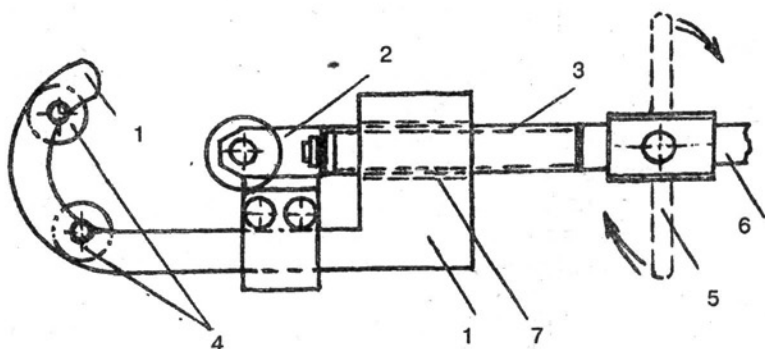
Рис. 68. Трехроликовый труборез:
