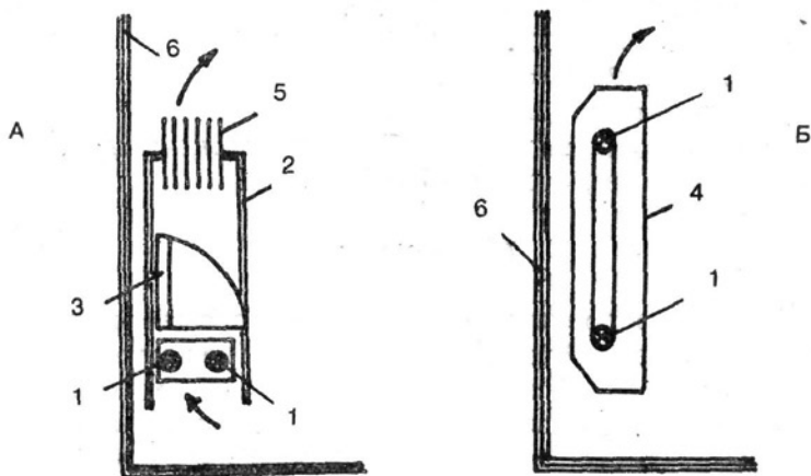
Рис. 34. Конвекторы:
