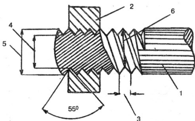
Рис. 62. Элементы резьбы:
