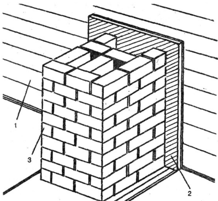
Рис. 82. Печь, имеющая закрытые поверхности, обращенные в отступки (пространство между печью и стеной):
