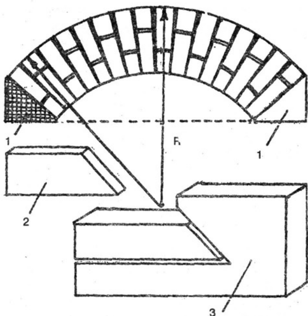
Рис. 91. Шаблоны для разметки пята: 1 - пята; 2 - шаблон пята; 3 - обратный шаблон пята; Я - радиус арочной кладки
