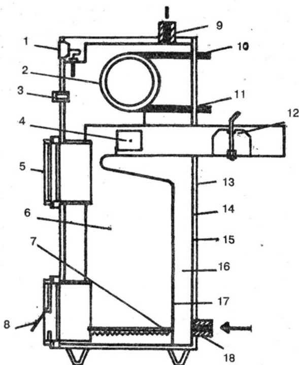
Рис. 21. Котел "Пламя":
