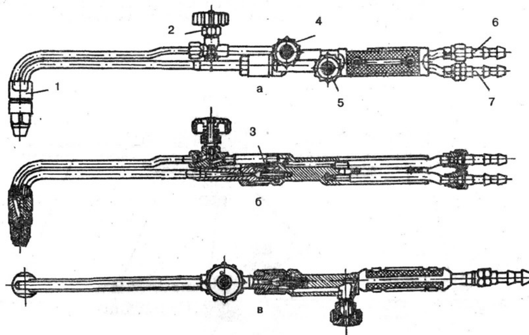
Рис. 67. Резак газовый:
