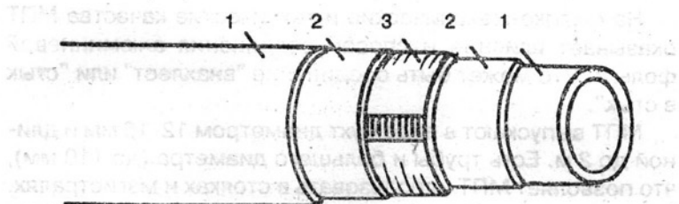
Рис. 44. Металлополимерная труба:
