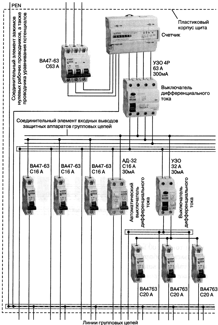
Рис. 3.14. Пример схемы группового распределительного щита
