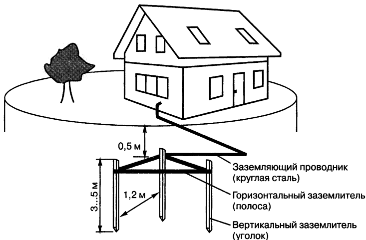
Рис. 4.10. Система заземления, подведенная к дому
