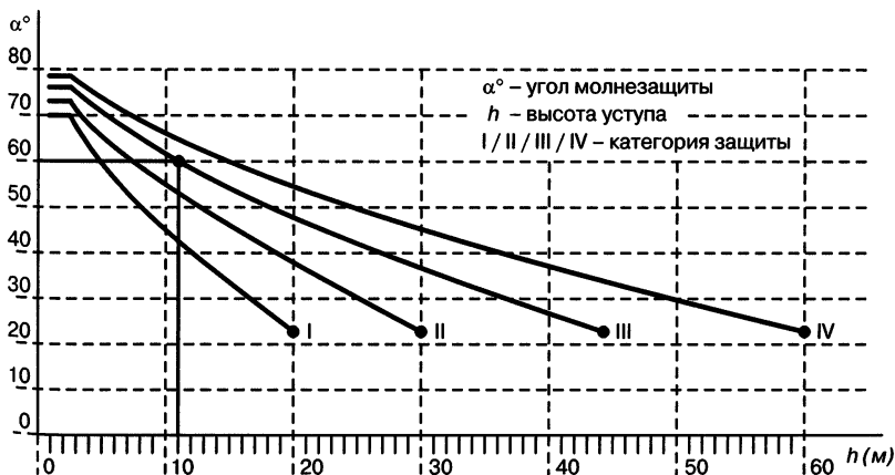
Рис. 6.3. График зависимости радиуса зоны защиты от высоты дома
