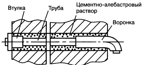
Рис. 4.2. Конструкция для прохода стены при вводе в дом
