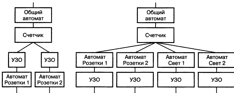
Рис. 4.7. Схемы включения УЗО
