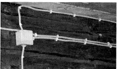
Рис. 4.19. Проводка открытым способом с использованием электротехнических скоб
