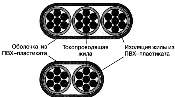
Рис. 5.1. Структура провода ПУНП
