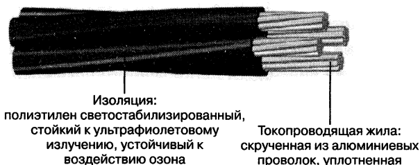
Рис. 4.4. Самонесущий изолированный провод СИП: конструкция
