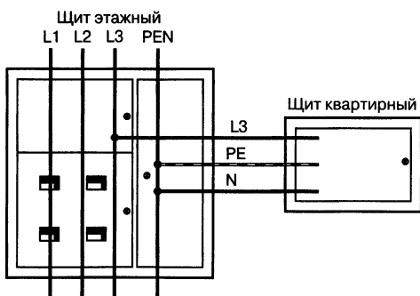
Рис. 2.9. Наглядное представление системы защитного заземления TN-C с незаконным локальным расщеплением PEN на этажном щитке
