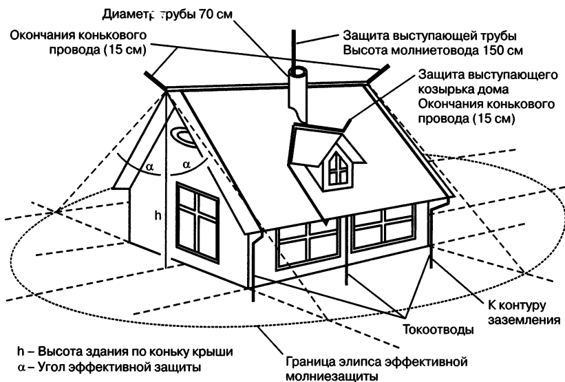
Рис. 6.2. Расчет эффективной зоны молниезащиты частного дома
