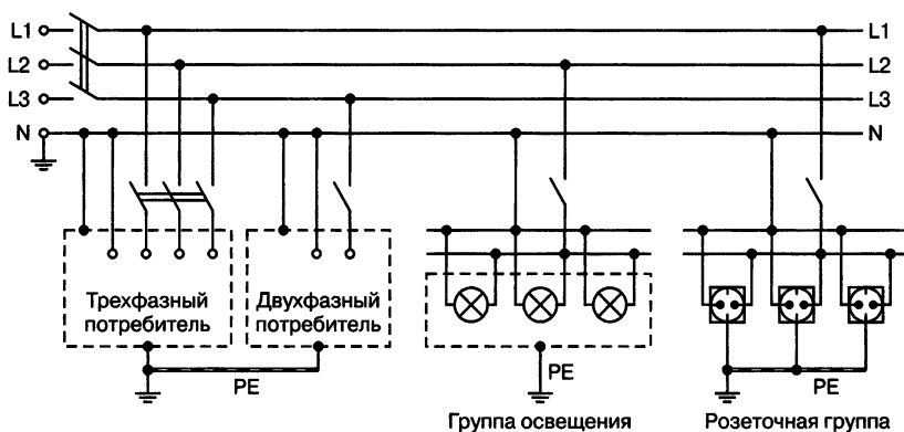
Рис. 2.6. Система с заземленной нейтралью TT
