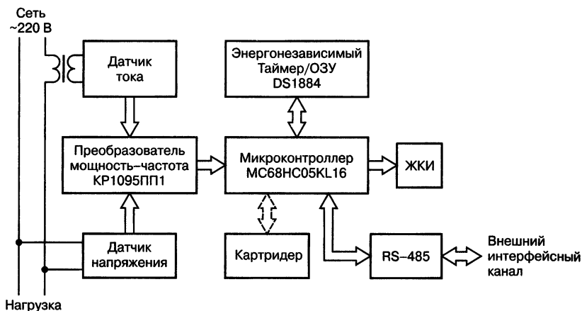
Рис. 10.6. Блок-схема многотарифного электронного однофазного электросчетчика
