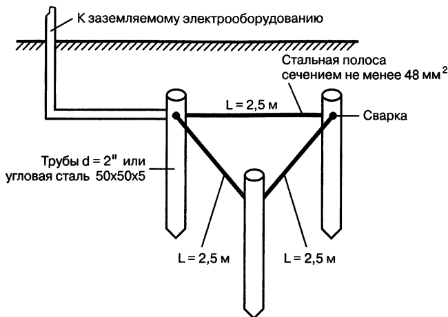
Рис. 4.9. Подземная часть системы заземления
