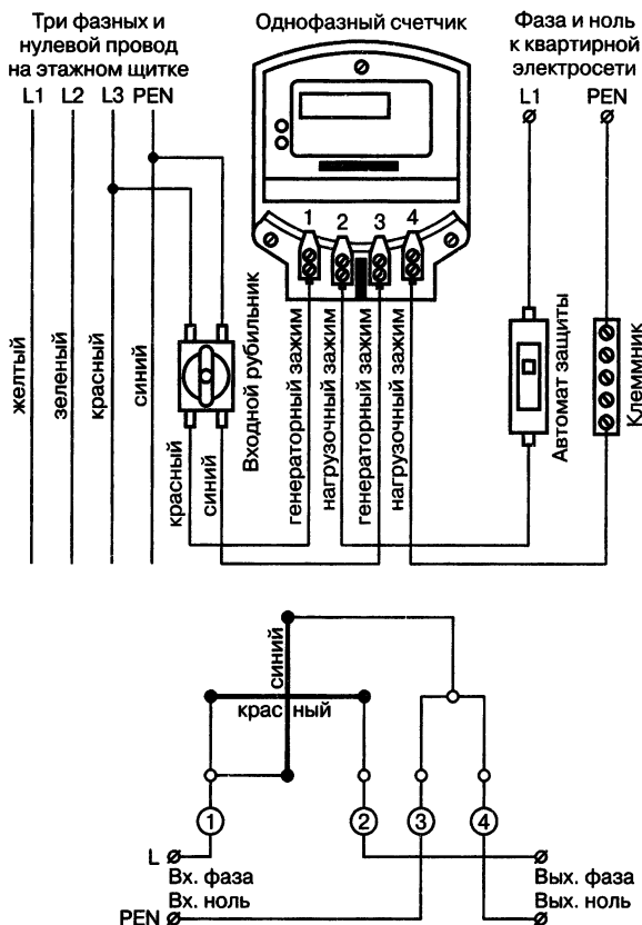
Рис. 10.10. Демонстрационная схема подключения однофазного электросчетчика
