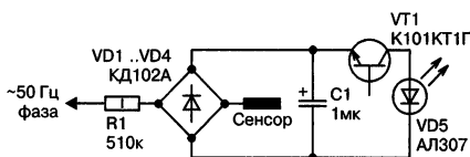
Рис. 11.12. Базовая схема индикатора фазового провода с сенсором на плече выпрямительного моста, выполненного на основе релаксационных генераторов на лавинных транзисторах
