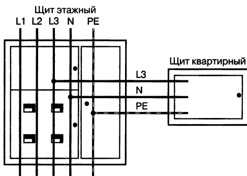
Рис. 2.10. Реализация системы защитного заземления TN-C-S при однофазном вводе в квартиру
