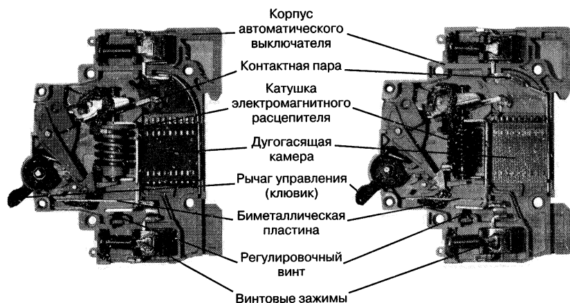
Рис. 8.1. Устройство автоматических выключателей
