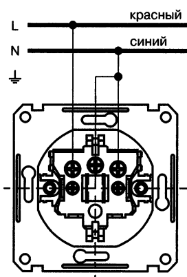
Рис. 11.2. Неправильное подключение заземляющего провода
