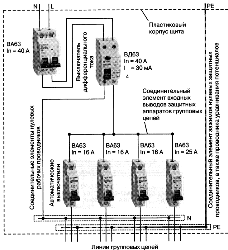
Рис. 3.13. Пример схемы квартирного группового распределительного щита
