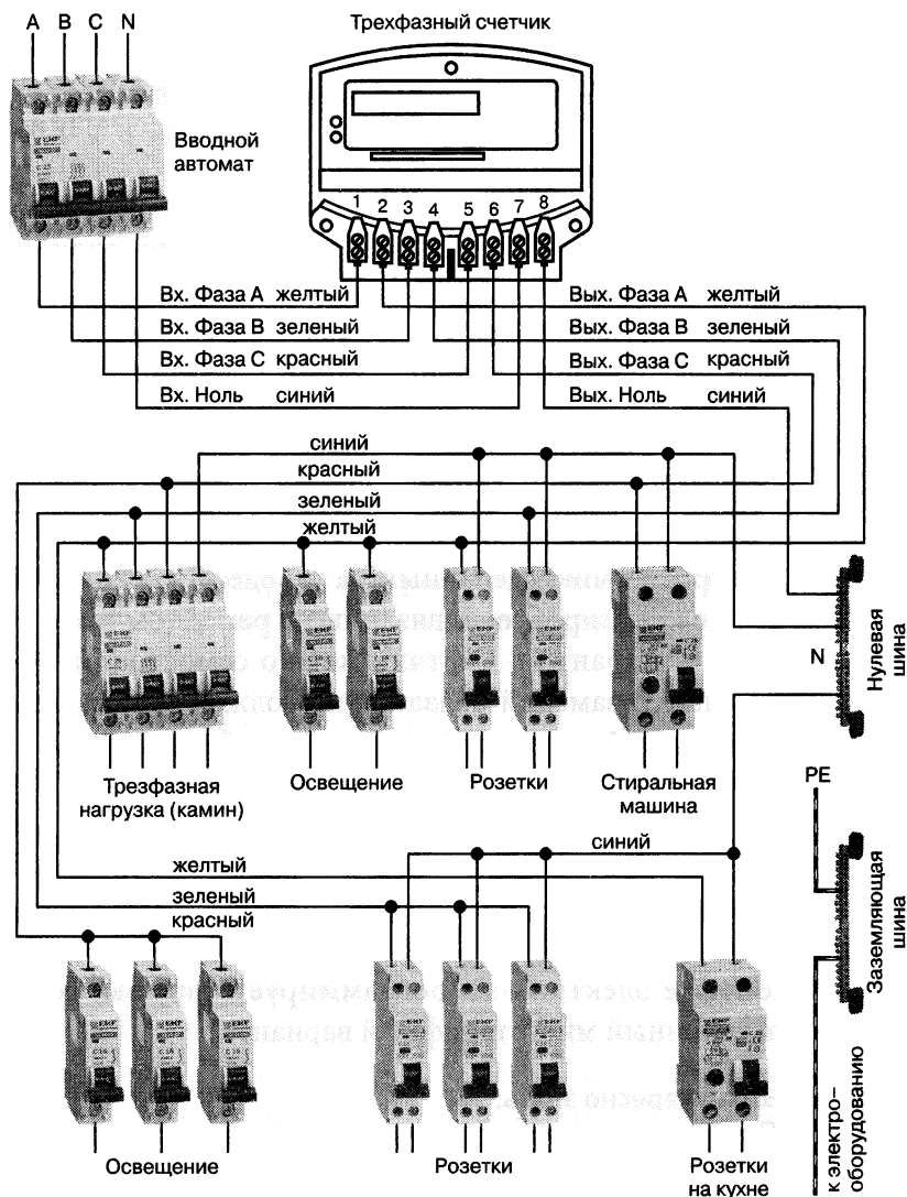
Рис. 10.13. Подключение трехфазного счетчика
