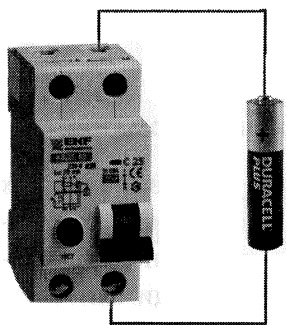
Рис. 9.8. Проверка электромеханического АДТ-63
