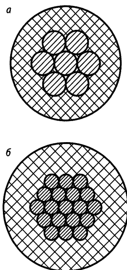
Рис. 5.2. Структура провода марки ПВ: а — провод ПВ1; б — провод ПВ3
