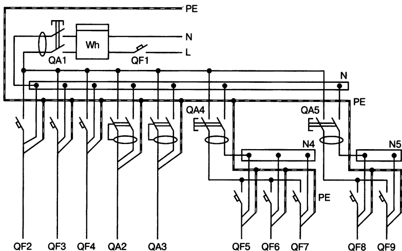
Рис. 3.9. Принципиальная схема квартирного щитка
