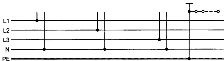
Рис. 3.6. Принципиальная схема щитков ЩЭМ3-4200 и ЩЭМ3-4201
