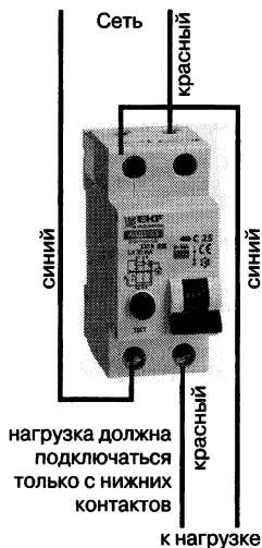
Рис. 9.14. Четвертая ошибка: нагрузка должна подключаться только с нижних контактов
