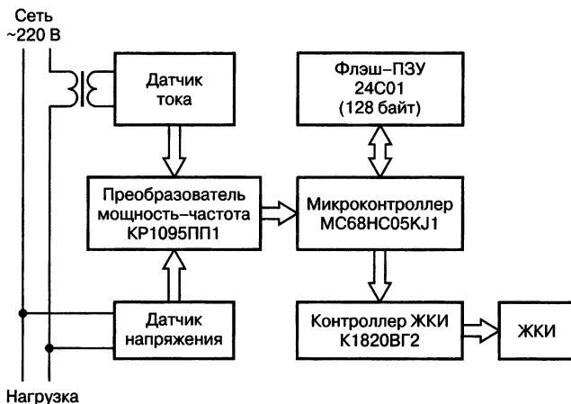
Рис. 10.5. Блок-схема простого электронного однофазного счетчика электроэнергии
