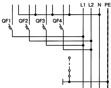
Рис. 3.7. Принципиальная схема щитка ЩЭ1409
