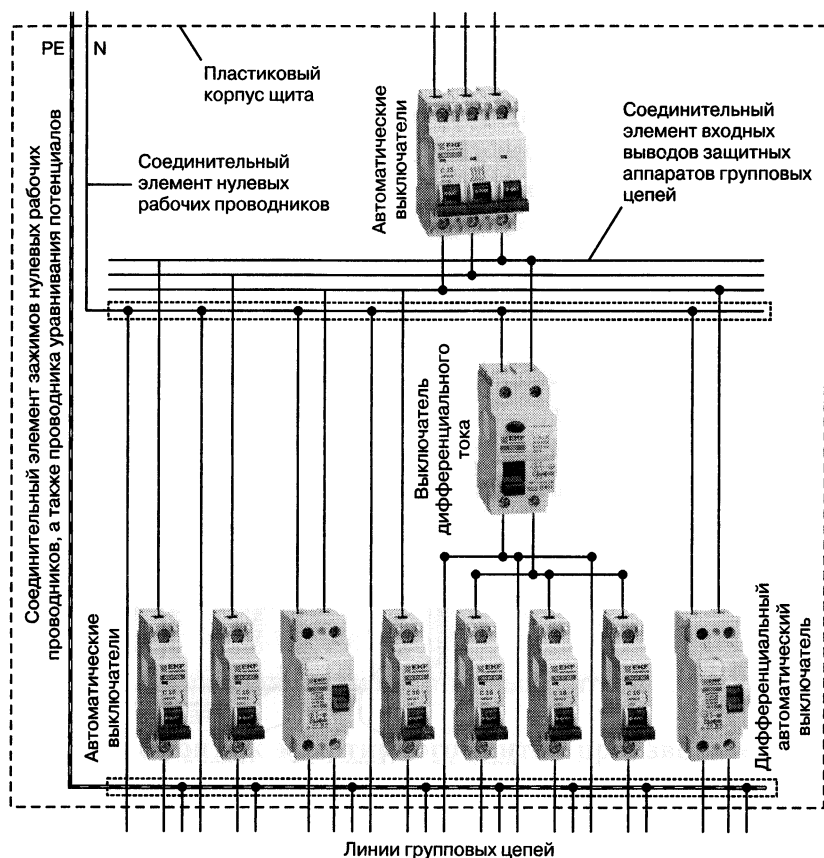
Рис. 3.12. Схема небольшого квартирного щита для многоквартирной квартиры
