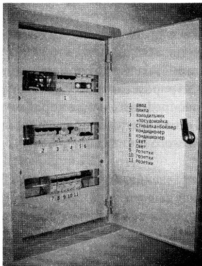
Рис. 3.8. Внешний вид квартирного щитка для скрытой установки
