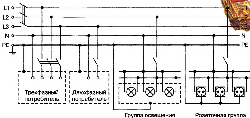
Рис. 2.4. Дорогостоящая система защитного заземления TN-S
