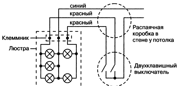
Рис. 11.3. Схема включения люстры с двухклавишным выключателем
