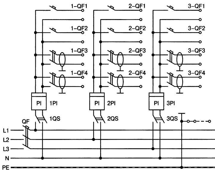
Рис. 3.5. Принципиальная схема щитков ЩЭМ3-4210 и ЩЭМ3-4211
