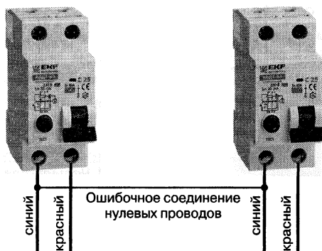
Рис. 9.11. Первая ошибка: соединение нулевых проводников, идущих через разные защитные устройства
