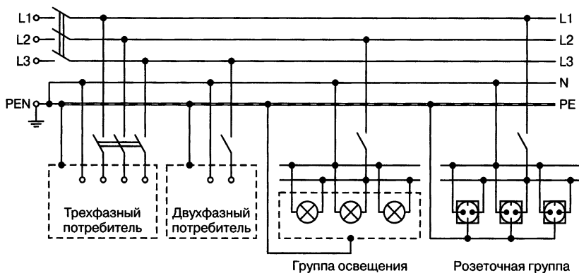
Рис. 2.5. Современная система защитного заземления TN-C-S
