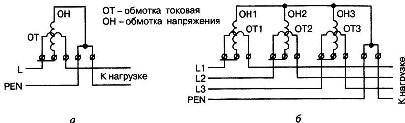
Рис. 10.9. Принципиальные схемы включения счетчиков: а — однофазного; б — трехфазного
