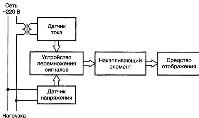
Рис. 10.3. Блок-схема однофазного индукционного счетчика
