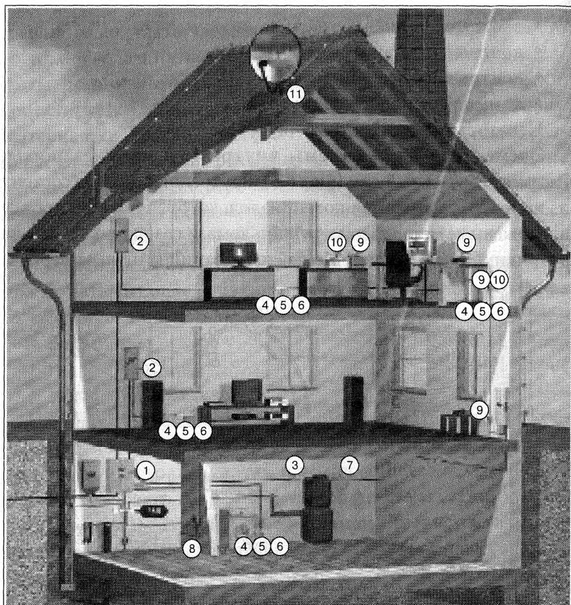
Рис. 6.6. Внутренняя система молниезащиты частного дома: 1–2 — устройства молниезащиты Lightning-Controllers и грозоразрядники; 3–6 — системы защиты электросетей; 7–10 — системы защиты информационных и связанных сетей
