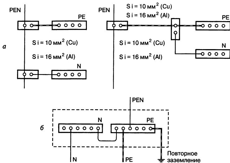
Рис. 2.3. Расщепления PEN проводника в ВПУ: а — схемы расщепления; — наглядное представление
