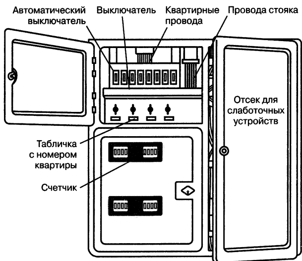
Рис. 3.3. Пример исполнения электрощкафа
