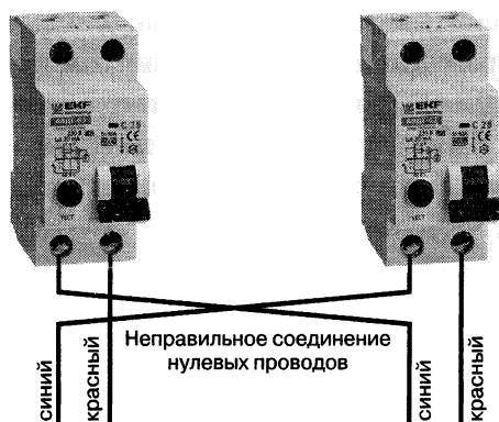
Рис. 9.12. Вторая ошибка: неправильное подключение проводников
