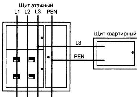
Рис. 2.8. Наглядно представление системы защитного заземления TN-C
