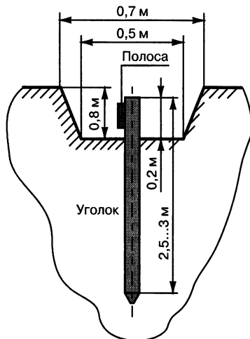
Рис. 4.8. Пример размещения вертикального заземлителя
