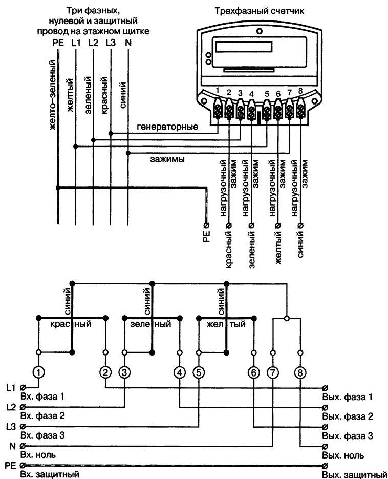
Рис. 10.11. Демонстрационная схема подключения трехфазного электросчетчика
