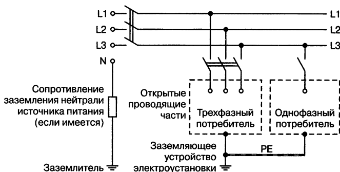
Рис. 2.7. Система с изолированной нейтралью IT
