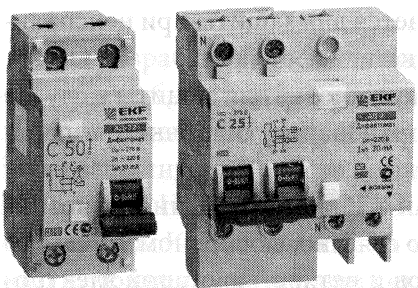
Рис. 9.5. Так выглядят автоматические выключатели дифференциального тока с электронным УЗО в комплекте
