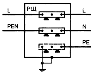
Рис. 4.14. Подключение дома к контуру заземления по системе TT
