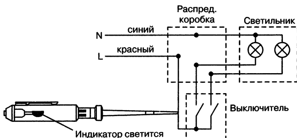
Рис. 11.4. Определение проводов
