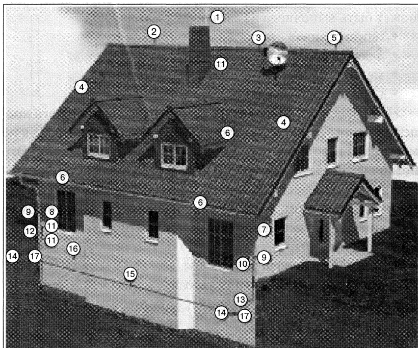
Рис. 6.4. Элементы внешней молниезащиты:
