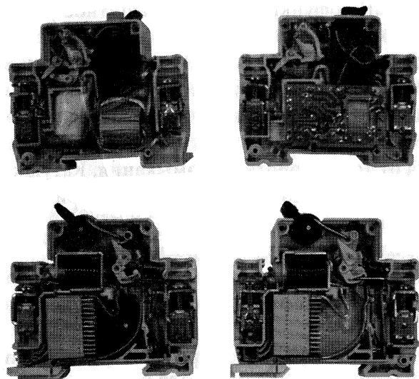
Рис. 9.3. Внутреннее устройство АВДТ-63 (левый — электромеханический, правый — электронный). С одной стороны — это УЗО, а если перевернуть, то с другой стороны — это уже автоматический выключатель. В комплексе же это АВДТ
