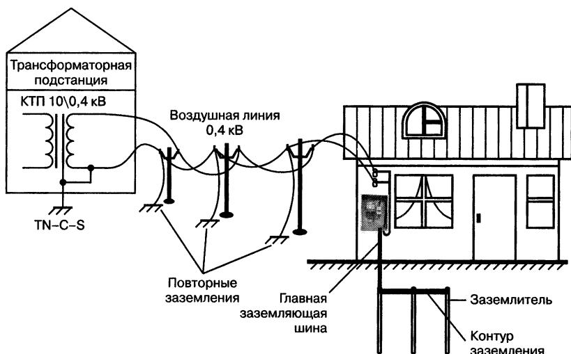
Рис. 4.12. Упрощенная схема подключения дома
