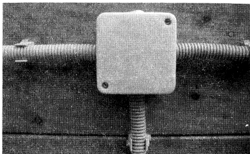
Рис. 4.22. Монтаж с использованием гофрированных трубок
