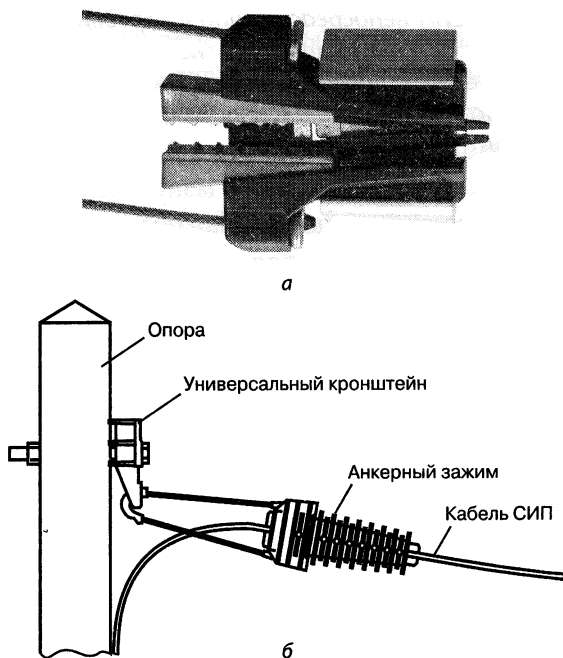
Рис. 4.5. Анкерные (клиновые) зажимы: а — устройство; б — пример применения
