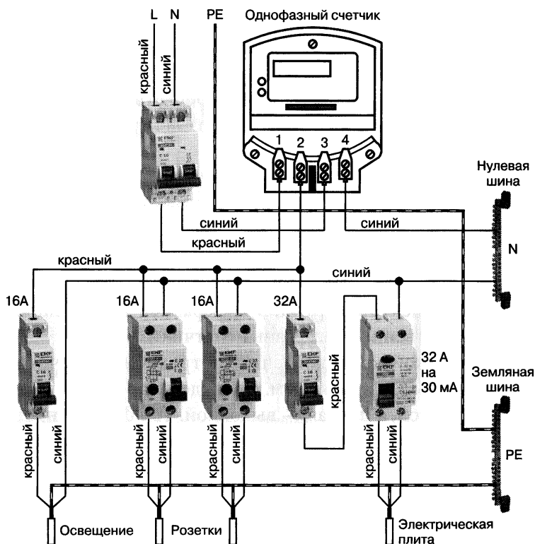
Рис. 10.12. Подключение однофазного счетчика
