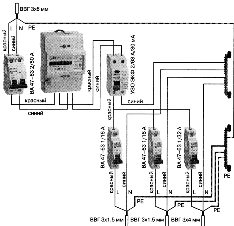
Рис. 3.11. Пример наглядной схемы простого квартирного щитка
