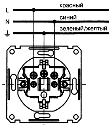
Рис. 11.1. Схема подключения розеток
