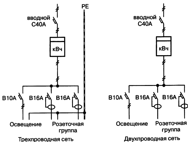
Рис. 9.10. Схемы подключения АВДТ
