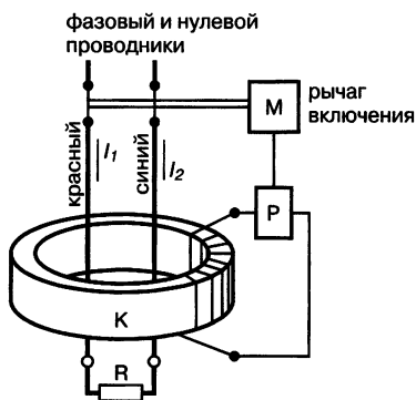
Рис. 9.1. Как работает УЗО: случай полной исправности электрооборудования и подводящих линий
