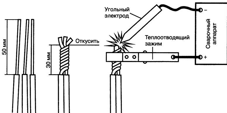
Рис. 11.6. Методы соединения: сварка
