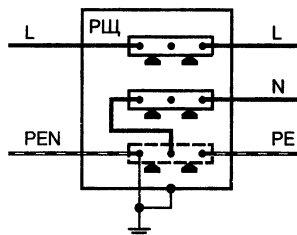
Рис. 4.13. Расщепление PEN проводника и преобразование системы TN-C на TN-C-S
