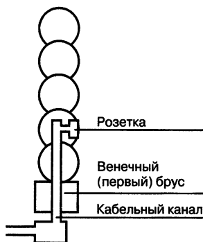
Рис. 4.25. Принцип создания скрытой проводки в доме из бревен
