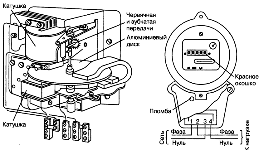
Рис. 10.4. Однофазный индукционный счетчик
