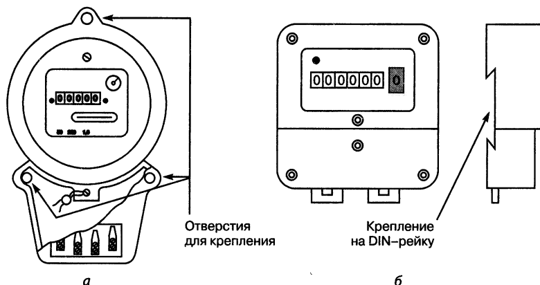
Рис. 10.7. Варианты крепления электросчетчиков: а — традиционное крепление на три шурупа; б — крепление на DIN-рейку
