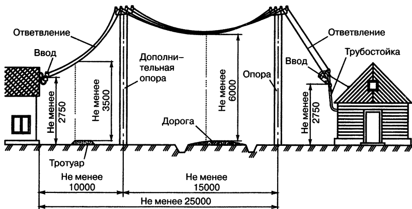
Рис. 4.1. Пример схемы отведений от воздушной линии 380 В и вводов в деревянные дома
