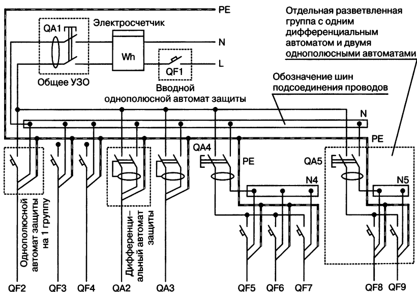
Рис. 3.10. Принципиальная схема квартирного щитка с комментариями
