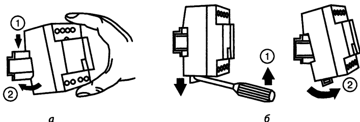
Рис. 3.15. Методика установки автомата на DIN-рейку
