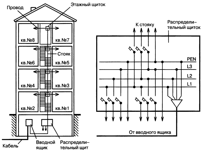
Рис. 3.1. Кабельный ввод в многоэтажный дом с системой заземления TN-C
