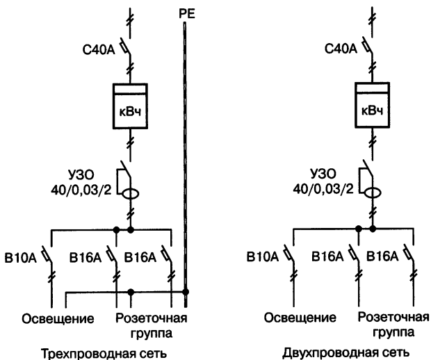
Рис. 9.9. Схемы включения УЗО
