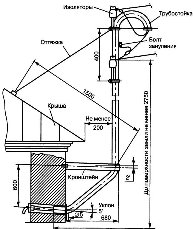
Рис. 4.3. Ввод в дом с использованием трубостойки
