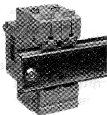
Рис. 3.16. Способ крепления автомата на DIN-рейке (вид со стороны рейки)
