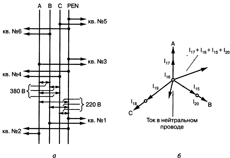
Рис. 3.2. Распределение нагрузки между фазами: а — структура электроснабжения стояка; б — ток в нейтральном проводе
