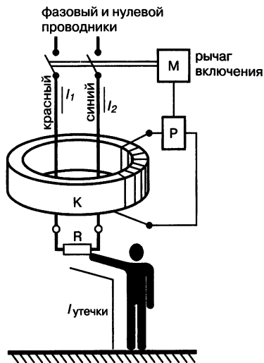
Рис. 9.2. Действие УЗО при возникновении тока утечки
