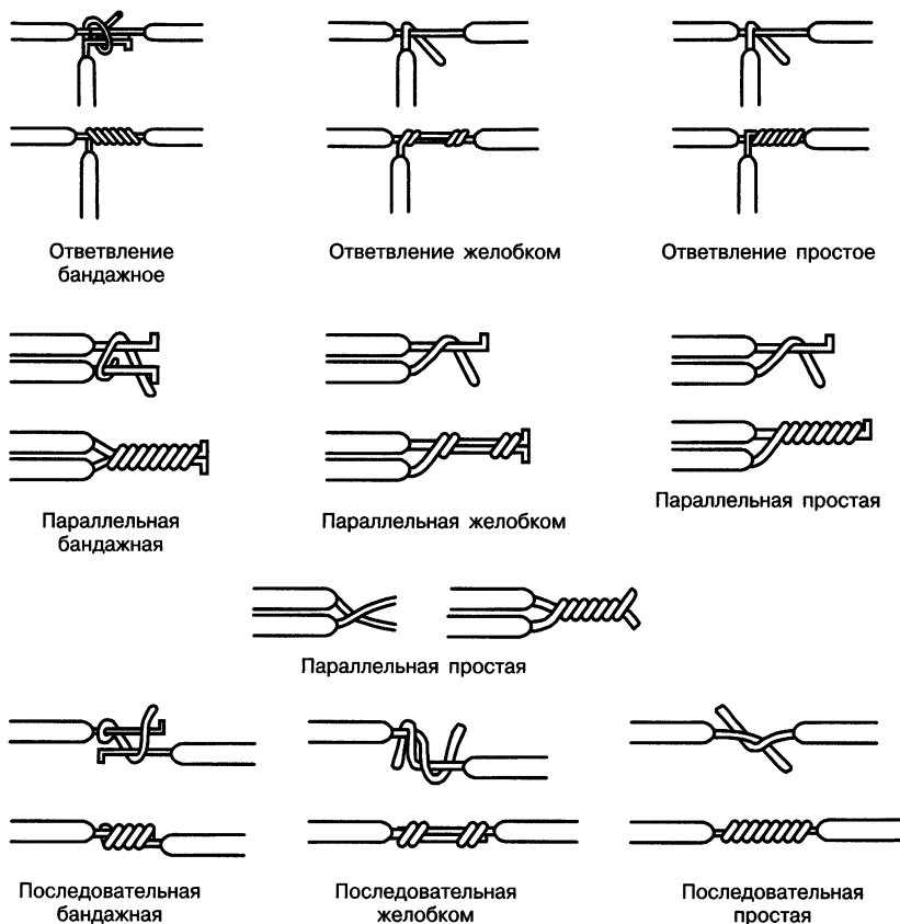
Рис. 11.7. Методы соединения: пайка
