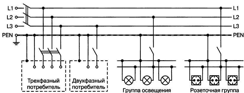
Рис. 2.2. Устаревшая система защитного заземления TN-C
