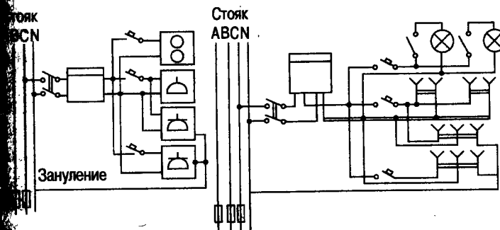
Схема квартирной групповой сети и ее присоединение к стояку
