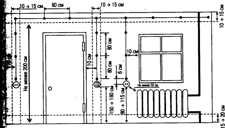
Рисунок 14. Нормативы, действующие при разметке проводки
