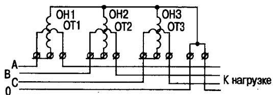
Рисунок 30. Схемы включения счетчиков
