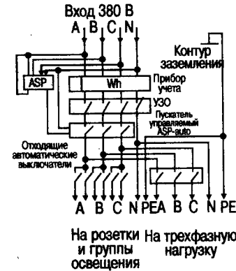
Рисунок 45. Рекомендуемые схемы включения (окончание)
