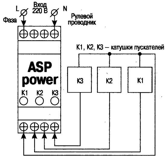
Рисунок 46. Схема подключения к электросети
