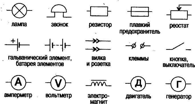
Рисунок 1. Общепринятые обозначения наиболее распространенных элементов электрической цепи
